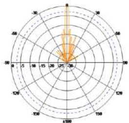
V-Pol Elevation
